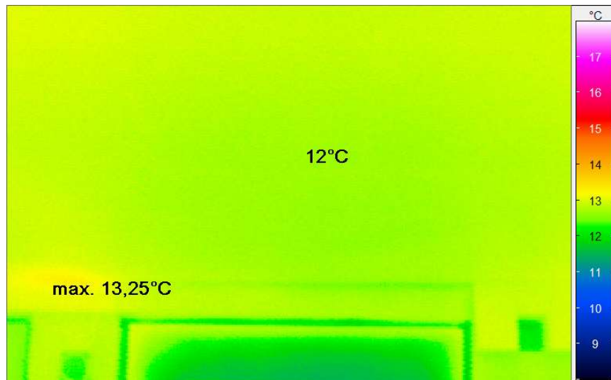
Abbildung 70: Die Thermographie der Unterseite der Kellerdecke (hier im nordwestlichen Kellerraum) zeigt ebenfalls sehr homogene Temperaturen, hier um 12°C. Die Deckenuntersicht ist durch eine armierte Spachtelung auf der Dämmplatte der Kellerdeckendämmung (von unten) gegeben. Diese Spachtelung weist nach Sichtkontrolle im gesamten Keller keine Veränderung gegenüber dem Neuzustand auf. Die leichte Temperaturerhöhung an der linken Bildseite rührt von dem dort durch die Dämmung durchtretenden Zuluftrohr (Wickelfalzrohr aus Stahlblech) her; die Zuluft hat eine Temperatur von um 19°C. Der Wärmeverlust durch die Kellerdecke beträgt im Mittel etwa 1,1 W/m 2 zum Zeitpunkt der Messung.
