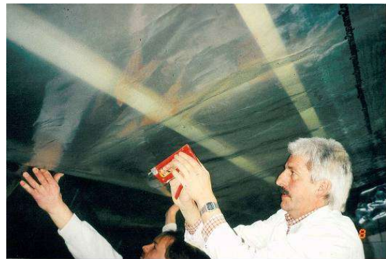
Abbildung 39: Anbringung der Luftdichtheitsbahn
