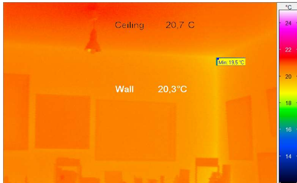
Abbildung 75: Die Innenthermographie der Northwest-Außenwanddecke im EG zeigt erwartungsgemäß die geometrische Wärmebrückenwirkung. Wegen des sehr geringen Wand-U-Wertes von 0,137 \text{ W}/(\text{m}^2\text{K}) sinkt die Temperatur allerdings auch in der Kante nicht unter 19,5 \text{ °C} ab. Die Temperatur an der Decke liegt nur wenig über der der Außenwand ( 20,3 \text{ °C} ), die Raumtemperaturschichtung ist somit gering. Alle Ergebnisse der Thermographie der Außenwände zeigen keine Auffälligkeiten und geben die nach der mehrdimensionalen Berechnung der Temperaturfelder bestimmten Projektierungswerte wieder (beachte: Die Deckenlampe ist nicht in Betrieb und nimmt daher Werte im Bereich der Raumtemperatur an).
