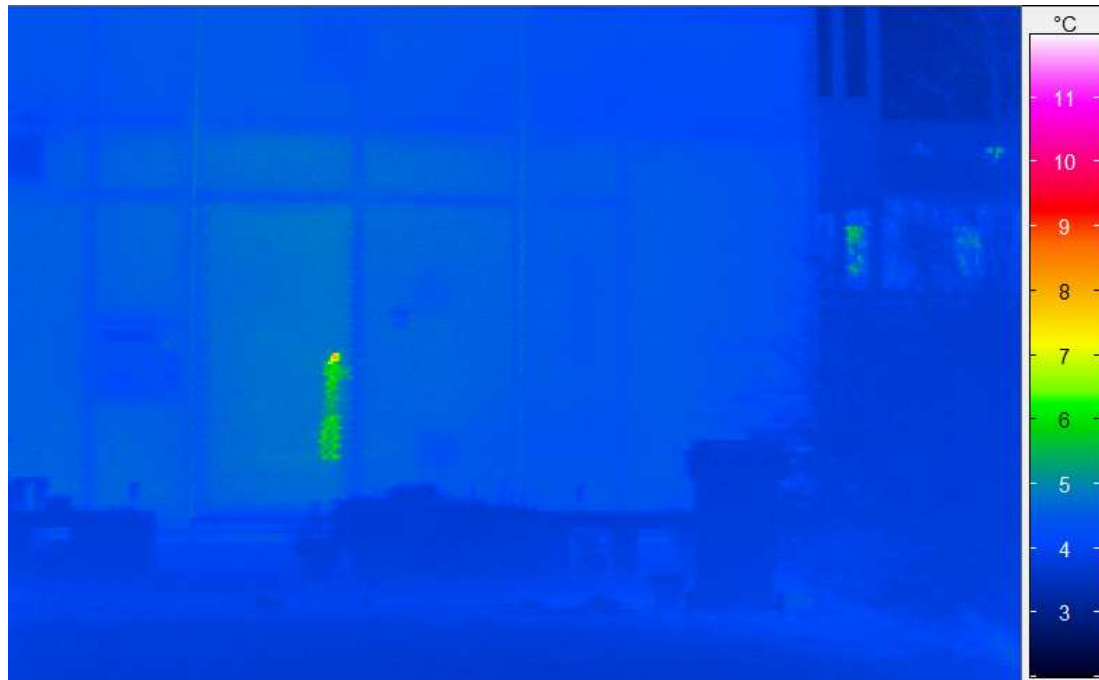
Abbildung 59: Die Aufnahme zeigt das Erdgeschoss und den unteren Teil des Obergeschosses des nördlichen Glasvorbaus, Northwestseite (01.01.2016). Auf der rechten Seite im Hintergrund sind Nachbargebäude, im Vordergrund Blumenkrüge und eine Mülltonne (Oberflächentemperatur 3,8 °C) zu erkennen. Die Glas-Außenoberfläche erscheint geringfügig wärmer (4,4 °C), dies ist eine Folge von drei etwa gleichermaßen beitragenden Effekten: 1) Die Emissivität (Abstrahlvermögen) von Glas ist etwas geringer als das der meisten anderen Oberflächen 2) Diese Oberfläche reflektiert vor allem Wärmestrahlung von Nachbargebäuden, die leicht höhere Oberflächentemperaturen haben 3) aufgrund von thermischer Trägheit ist es im Glasvorbau in der Frühe (immer noch vom Vortag) etwas wärmer als in der Außenumgebung. Auffällig ist hier allein das thermische Reflexionsbild des Thermographen. (links leicht unterhalb der Bildmitte).
