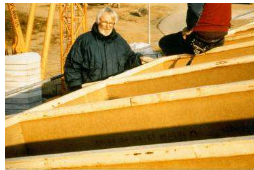
Abbildung 37: Dach während der Zimmermanns-Konstruktion. Im Bild auch Architekt Westermeyer. Gut erkennbar die Doppel-T-Träger aus Holz.
