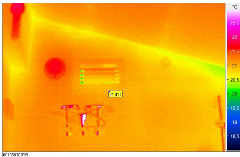
Abbildung 84: Duschbad im DG; die Temperatur im Raum beträgt etwa 21,6 °C; die Außenwand (nach Westen gerichtet) ist mit 21°C an der Oberfläche nur unwesentlich kühler. Dagegen ist die Raumlufttemperatur – ablesbar am Abluftventil, das stark umströmt wird – mit um 22°C etwas wärmer. In den verchromten Armaturen erkennt man teilweise verzerrte Reflexe des Thermographen. Die geometrische Wärmebrücke am Anschluss Wand/Dach ist deutlich ablesbar, jedoch sinken auch dort die Temperaturen nicht unter 20,6°C. Beachte: Das Licht (Energiesparlampe) war bewusst nicht eingeschaltet; die Lampe würde sonst deutlich mit einer sehr viel höheren Temperatur hervortreten (oben links). Im visuellen Bild ist daher der Reflex des Blitzes der visuellen Kamera erkennbar. Unter den hier gegebenen Randbedingungen ist im Duschbad auch bei lang anhaltenden hohen Raumluftfeuchten kein Kondensat und daher auch keine Schimmelbildung zu erwarten.
