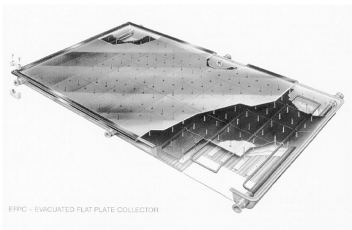
Abbildung 12: Der thermische Flachkollektor wurde auf dem Dach des Passivhauses aufgeständert. Verwendet wurden auf etwa 50 mbar evakuierte Flachkollektoren (bei diesem Unterdruck ist Konvektion im Füllgas (Argon) praktisch unterdrückt; es bleibt der Wärmeverlust durch Wärmeleitung).
