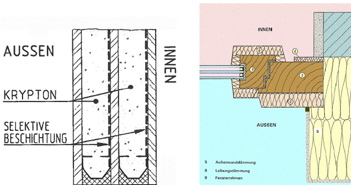
Abbildung 94: Links: Die verwendete Dreifach-Wärmeschutzverglasung mit drei Scheiben im schematischen Aufbau.
