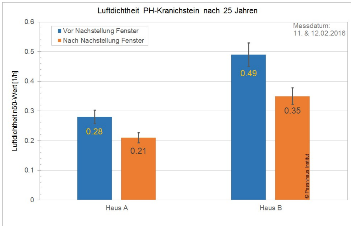
Abbildung 126: Luftdichtheitsmessungen im Februar 2016 vom Passivhaus Kranichstein (Haus A und B) vor und nach dem Austausch der Fenster- und Türendichtungen nach 25 Jahren.
