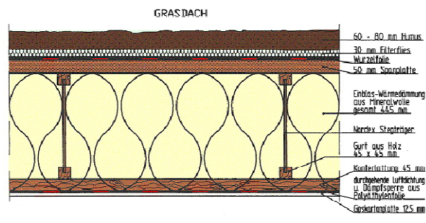
Abbildung 36: Der Dachaufbau im Passivhaus Darmstadt Kranichstein. Der Grasdachaufbau liegt auf einer von Stegträgern abgetragenen Spanplatte. Der Achsabstand der Stegträger konnte mit 1,08 m relativ hoch gewählt werden. Zum Raum hin folgt eine Konterlattung (45 mm), die durchgehende Luft- und Dampfdichtung (Polyethylenfolie) und eine Gipskartonplatte. Bei 445 mm Dämmstoffdicke ergibt sich ein Dach-U-Wert mit < 0,1 \text{ W}/(\text{m}^2\text{K}) .
