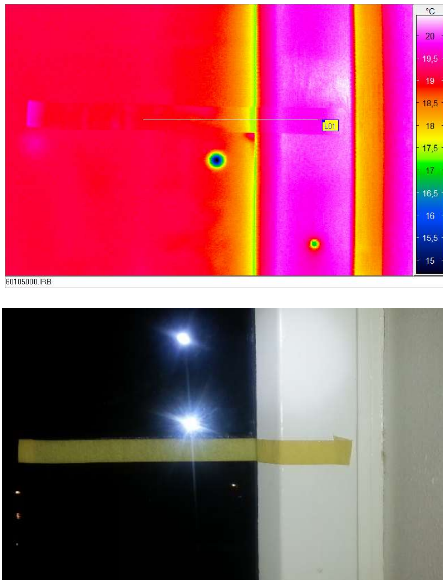
Abbildung 106: Innenthermographie mit hoher Temperaturauflösung von Verglasung, Fenster-rahmen und Fensteranschluss im Obergeschoss und zugehöriges Lichtbild (unten). Das aufgeklebte Kreppband dient wieder zur ungestörten Bestimmung der Oberflächentemperaturen.
