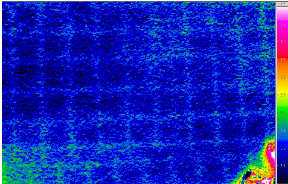
Abbildung 61: Bei extrem hoher Temperrauflösung sind im Detail der Außenwand die Schwalbenschwanz-Rillen in den EPS-Dämmplatten (die der Verkrallung des Putzes dienen) sichtbar. Dort sind durch die dickere Putzschicht der U-Wert etwas verringert und die Wärmekapazität etwas erhöht; der maximale Temperaturunterschied beträgt 0,2 Kelvin
