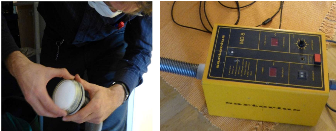
Abbildung 147: Filtrationssampler Typ MD 8 (Fa. Sartorius)
