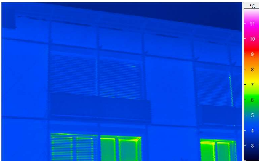
Abbildung 62: Anschluss Außenwand/Dach am First (vom 01.01.2016): Erwartungsgemäß fallen die äußeren Oberflächentemperaturen an der Kante leicht ab (Geometrie-effekt). Der deutlich dunklere Streifen ist allerdings ein Reflex des Himmels an der metallischen Dachrandeinfassung
