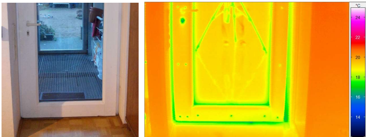
Abbildung 102: Haus-Eingangstür von innen als Foto (links) und als Thermogramm (rechts). In der Verglasung reflektieren das Stativ der Kamera und der Thermograph selber (Beine und Füße).
