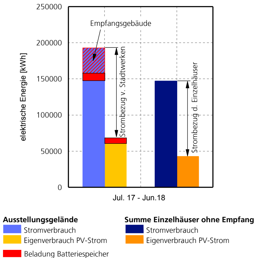
Bild 56: Gegenüberstellung von Stromverbrauch und Eigenverbrauch für die Einzelhäuser und das Ausstellungsgelände (FertighausWelt Wuppertal); Zeitraum Juli 2017 bis Juni 2018.
