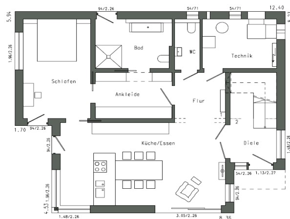
Erdgeschoss-Grundriss
