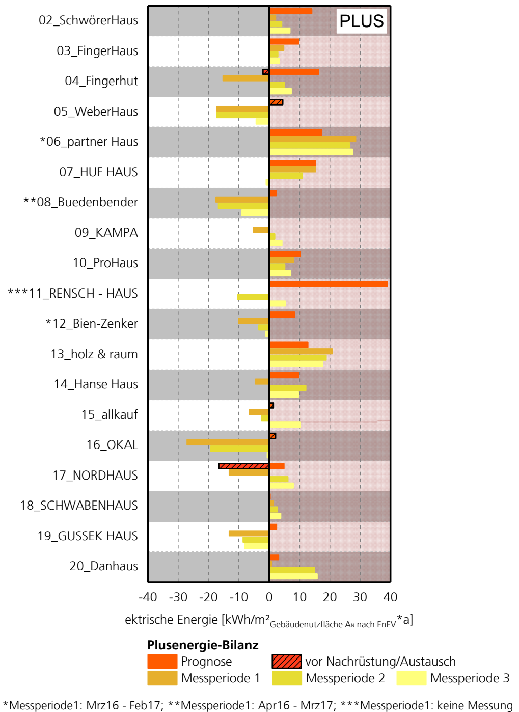
Bild 46: Plusenergiebilanz der Einzelhäuser, bezogen auf die Gebäudenutzfläche A N nach EnEV (FertighausWelt Wuppertal).
