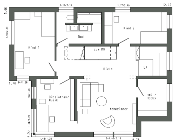
Obergeschoss-Grundriss
