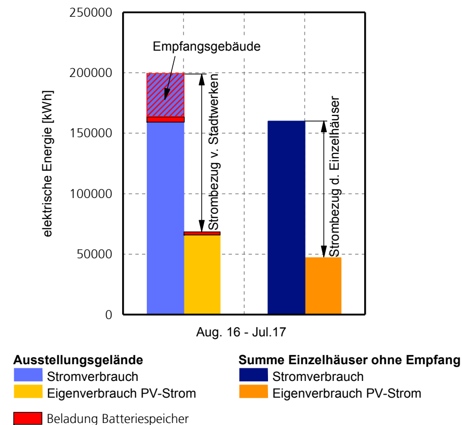
Bild 55: Gegenüberstellung von Stromverbrauch und Eigenverbrauch für die Einzelhäuser und das Ausstellungsgelände (FertighausWelt Wuppertal); Zeitraum August 2016 bis Juli 2017.
