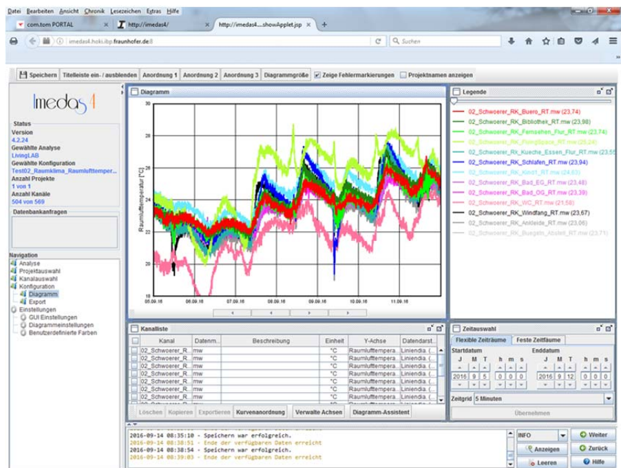
Bild 30: Imedas™-Auswerteoberfläche.
