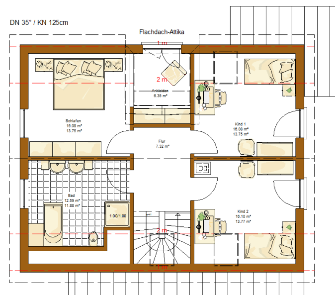
Dachgeschoss-Grundriss
