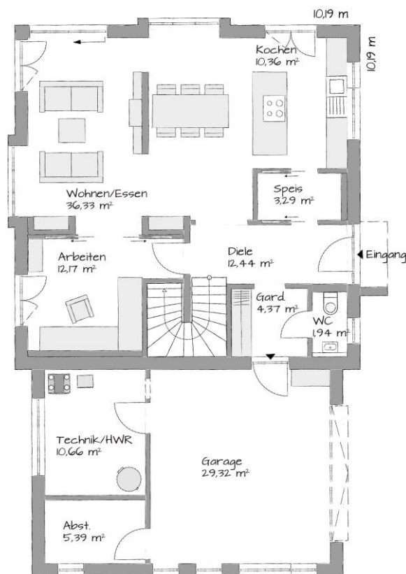
Erdgeschoss-Grundriss
