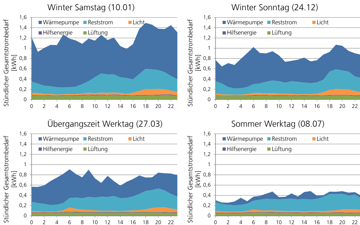
Bild 72: Stündlicher Verlauf der einzelnen Verbraucher für ein Musterhaus im Living Lab Wuppertal als Summenkurven an verschiedenen Tagen. Die deutlichen Unterschiede zwischen den Tagen sind hauptsächlich auf den Strombedarf der Wärmepumpe aufgrund der unterschiedlichen Außentemperaturen zurückzuführen.
