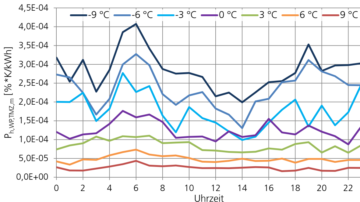
Bild 68: Verlauf des Effizienzhaus Plus-Wärmepumpen-Lastprofils bei unterschiedlichen Tagesmitteltemperaturen der Außenluft.
