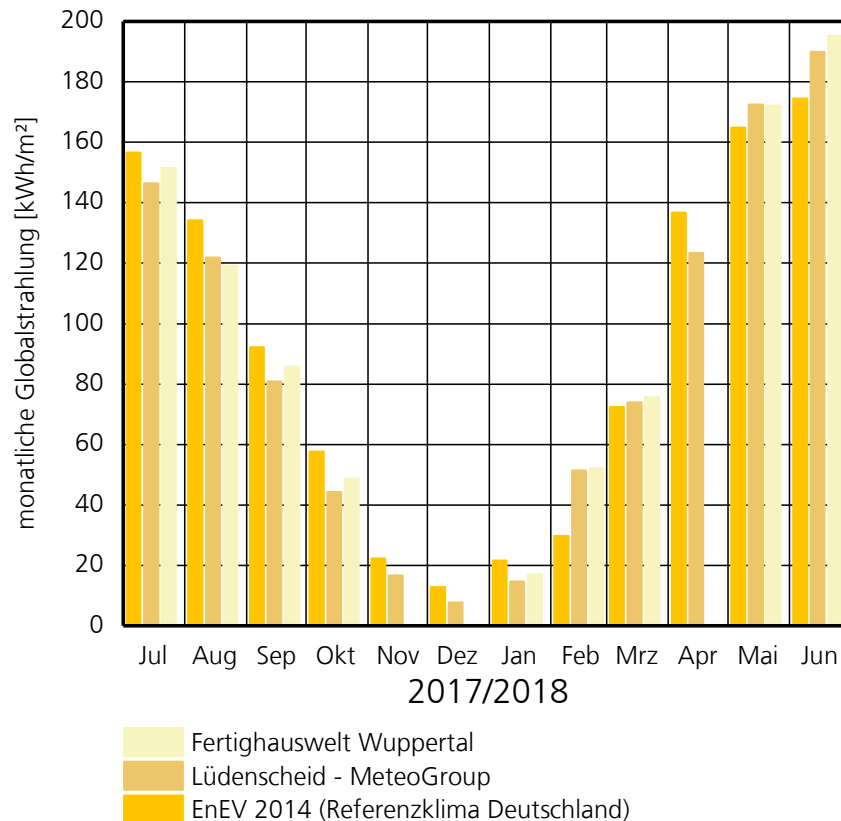
Bild 33: Monatsmittel der solaren Einstrahlung in Messperiode 3.
