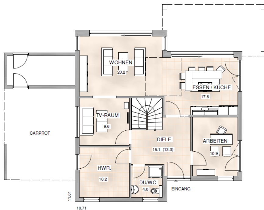
Erdgeschoss-Grundriss
