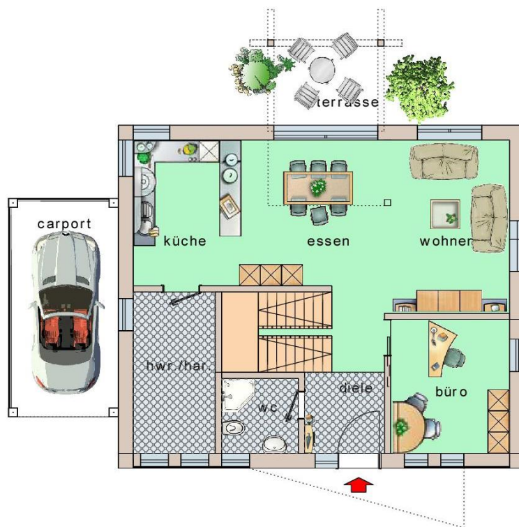
Erdgeschoss-Grundriss
