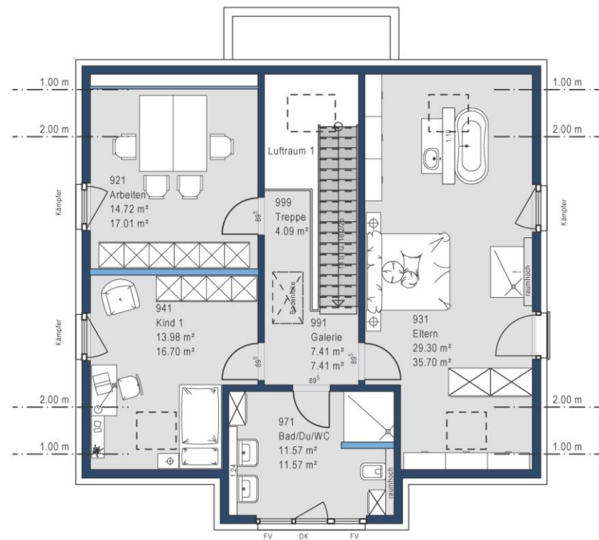
Obergeschoss-Grundriss
