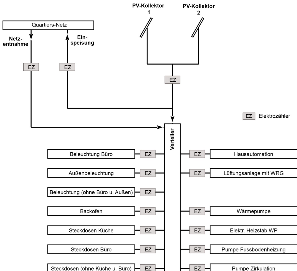
Bild 20: Messschema Elektroversorgung.
