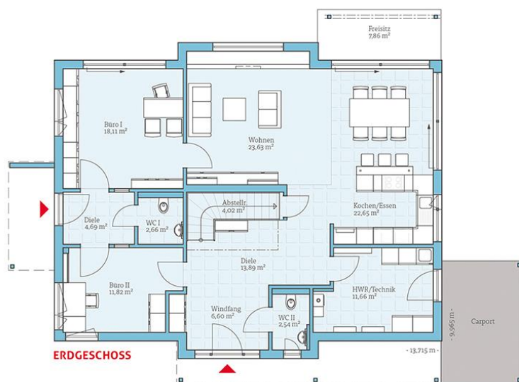
Erdgeschoss-Grundriss
