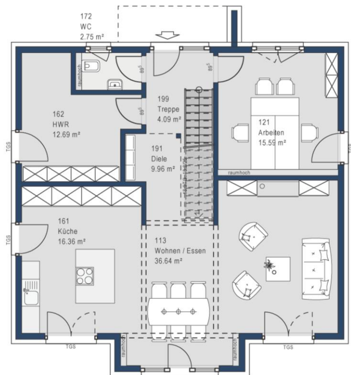
Erdgeschoss-Grundriss
