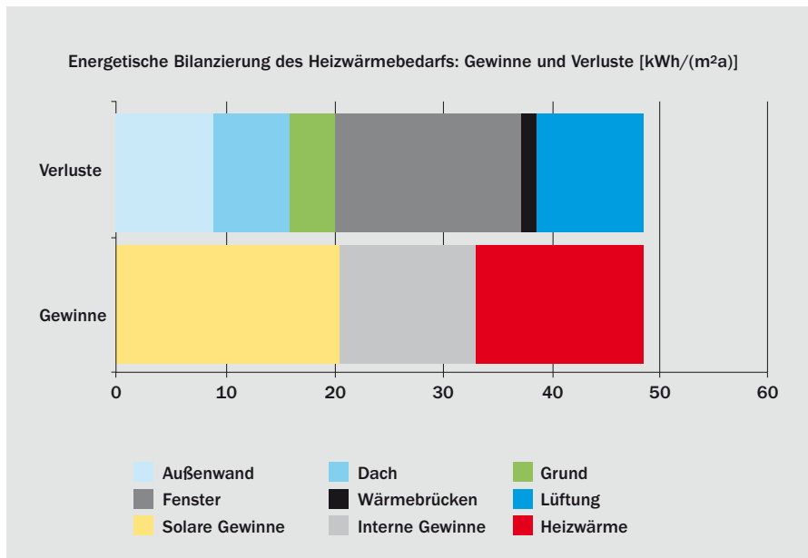
Jahres-Heizwärmebilanz für ein charakteristisches Passivhaus: Den Transmissionswärmeverlusten durch Wand, Grund, Dach, Fenster und Wärmebrücken und Lüftungswärmeverlusten stehen die nutzbaren Gewinne gegenüber: solare Gewinne, interne Wärme und der resultierende Heizwärmebedarf, der beim Passivhaus unter 15 kWh/(m²a) liegt.
