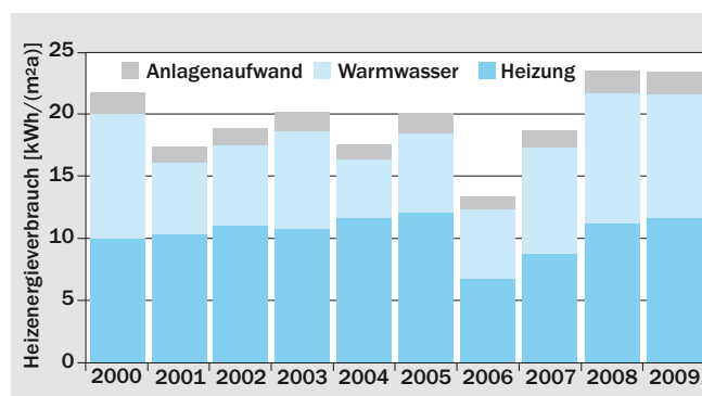
Heizenergieverbrauch von vier Doppelhaushälften (Mittelwert) in Passivbauweise in Nürnberg, Wachtelstraße
