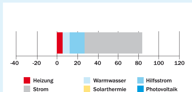
Primärenergiebilanz
